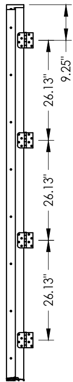
HINGE JAMB
